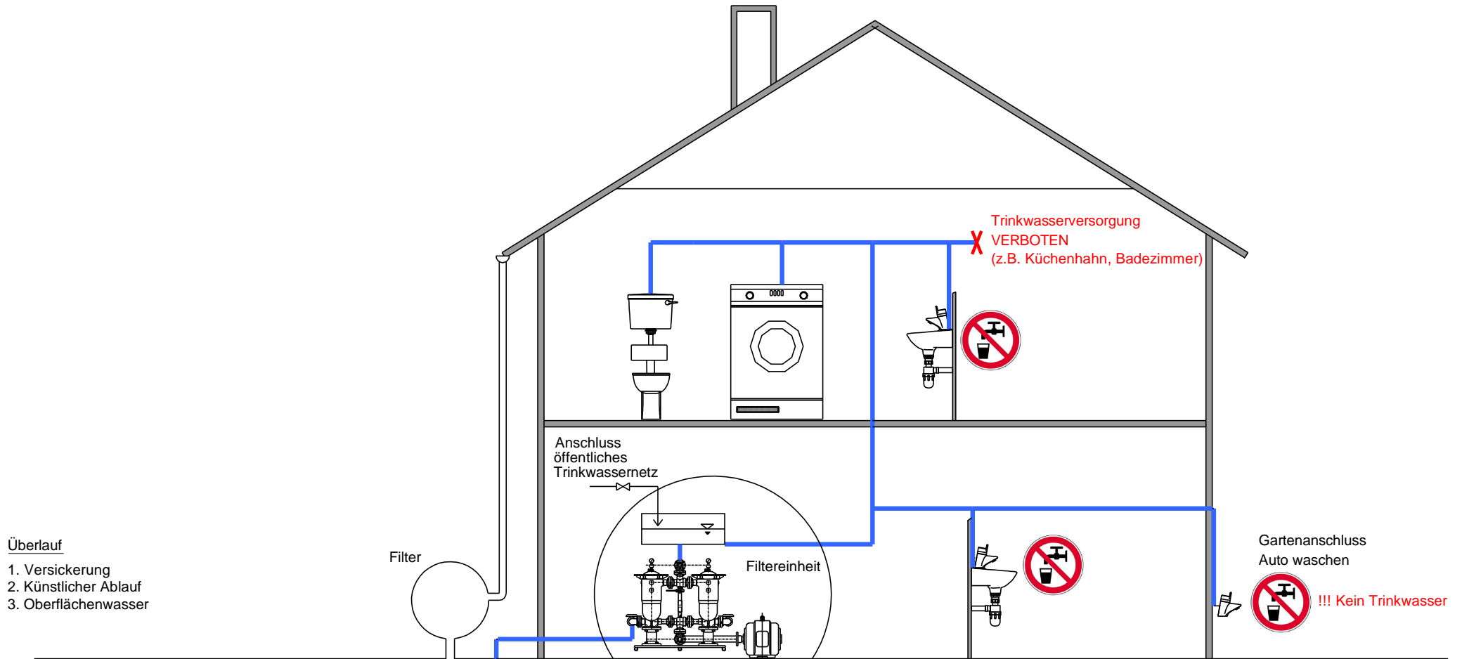
Beispiel Anschluss öffentliches Trinkwassernetz
