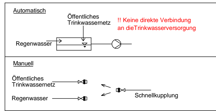
Beispiel Anschluss öffentliches Trinkwassernetz
